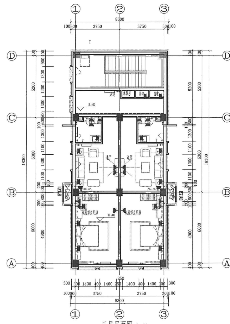
三层平面图 1:100
