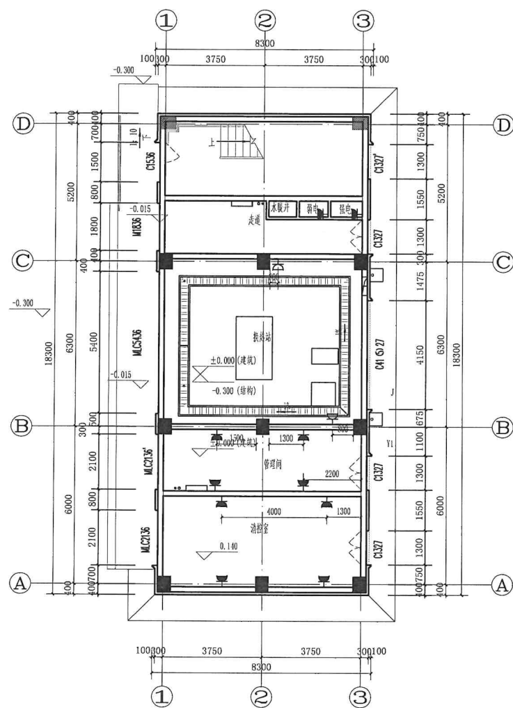
首层平面图 1:100
