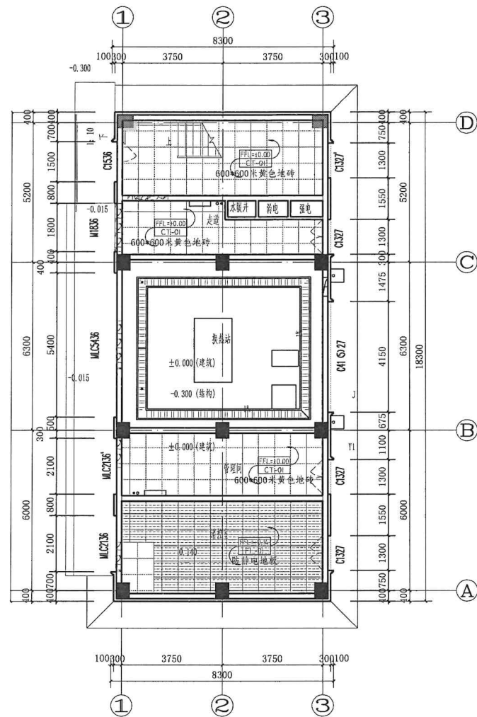
首层平面图 1:100
