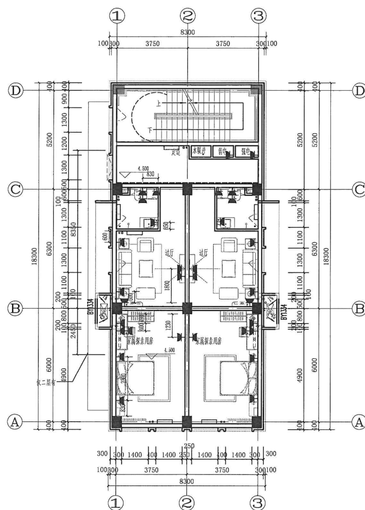
二层平面图 1:100
