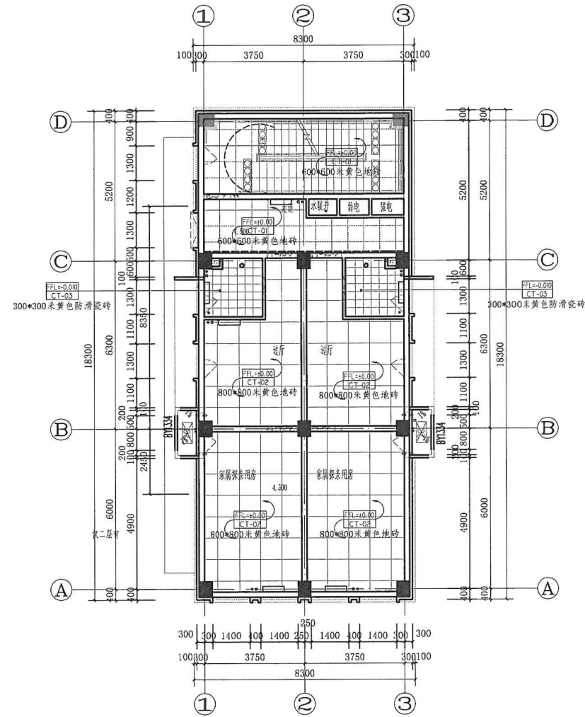
二层平面图 1:100
